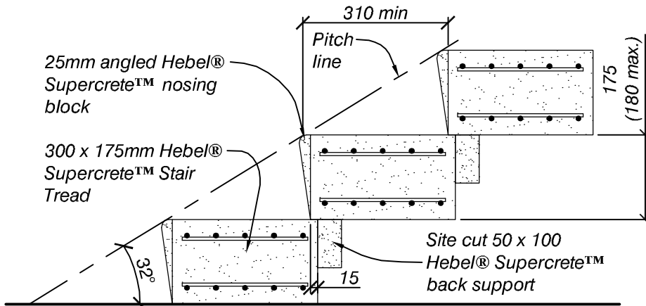
Accessible Stairway 32° max
